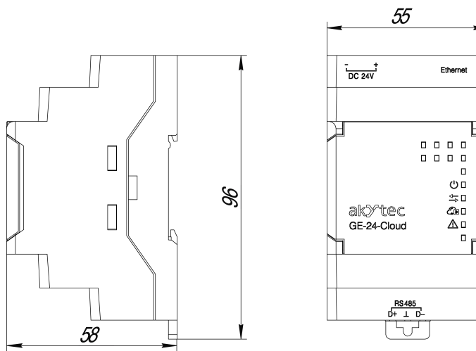
Abb. 1 Abmessungen
